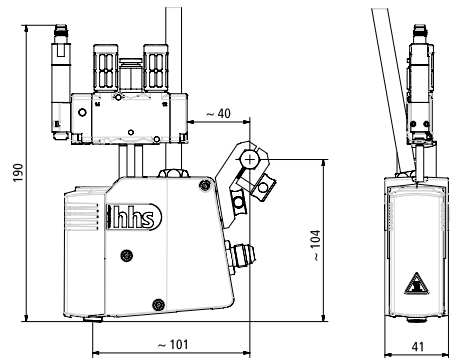
Technische Zeichnung
