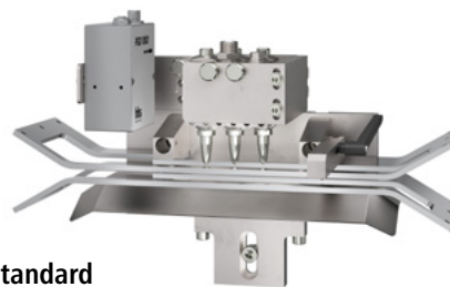
Inverto Die Alternative für den Klebstoffauftrag von oben und von unten
