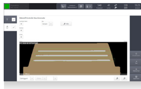
CorrBox Solution evo live Live Ansicht der Klebstoffüberwachung
