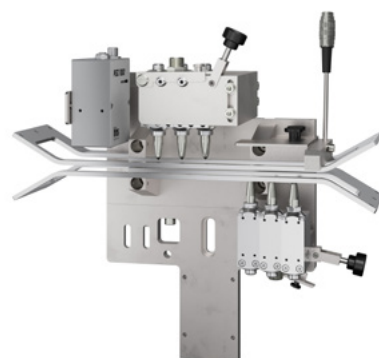
Inverto Die Alternative für den Klebstoffauftrag von oben und von unten
