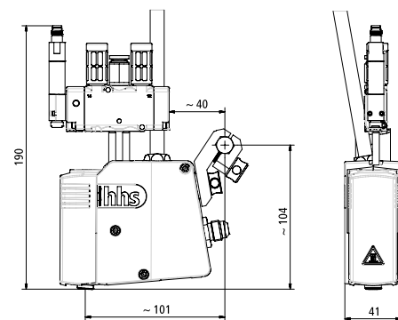
Dessin technique
